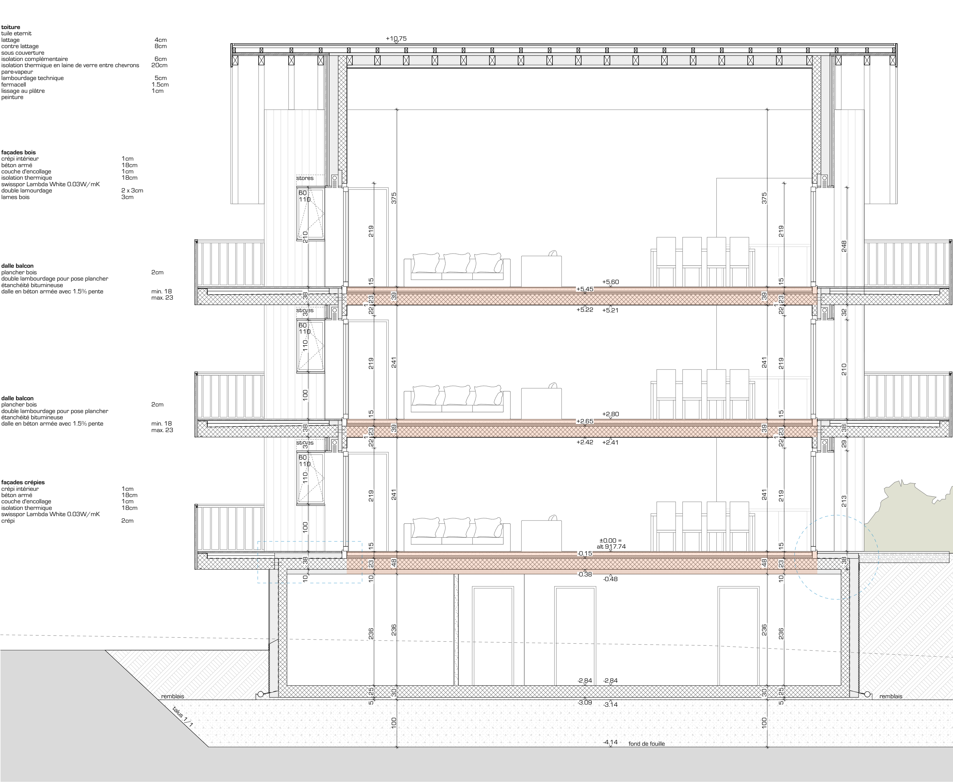
coupe DD
