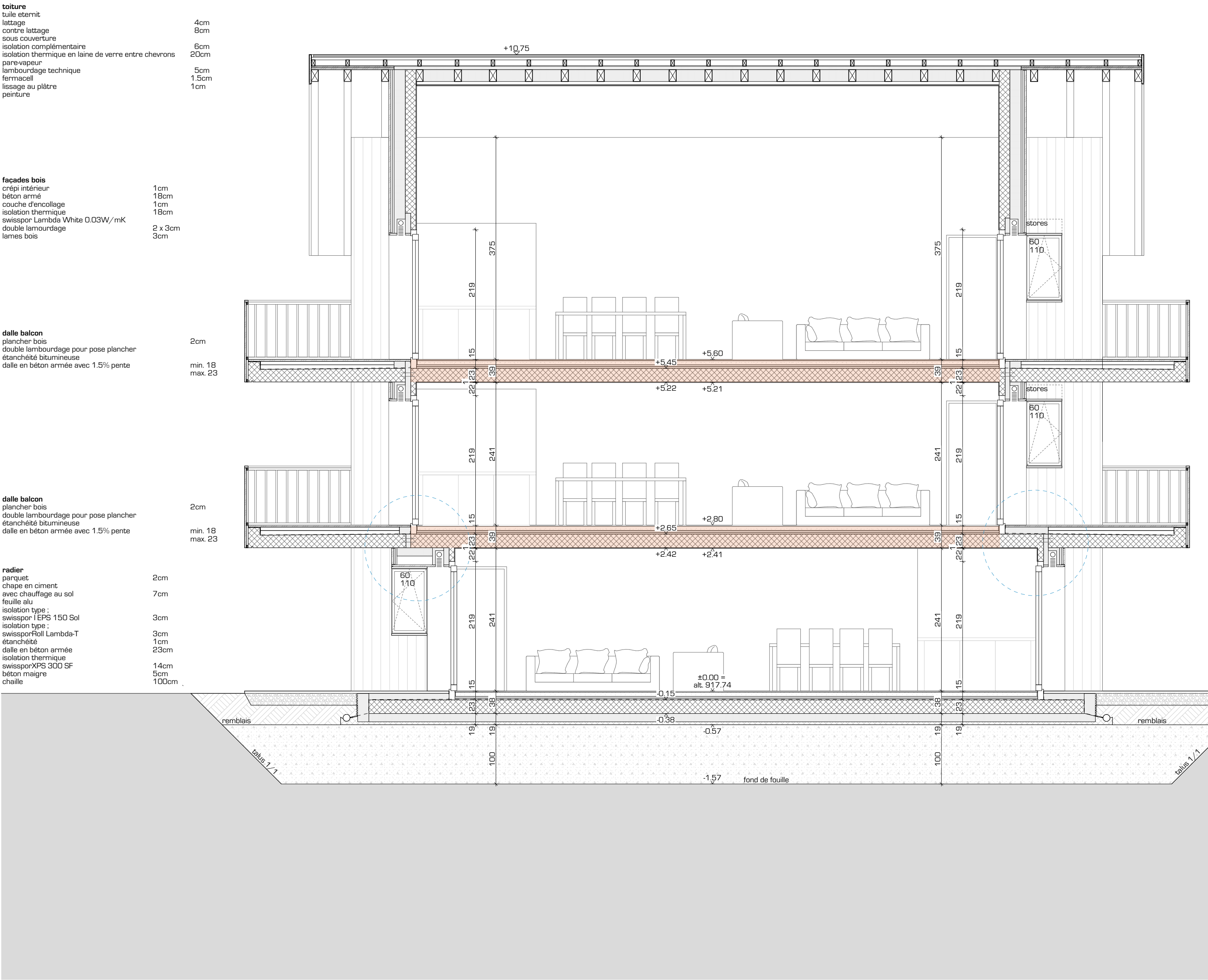
coupe EE
